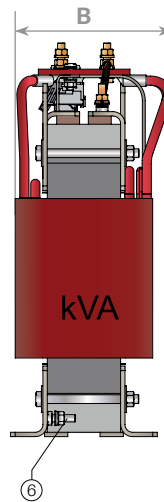
VISTA LATERAL
